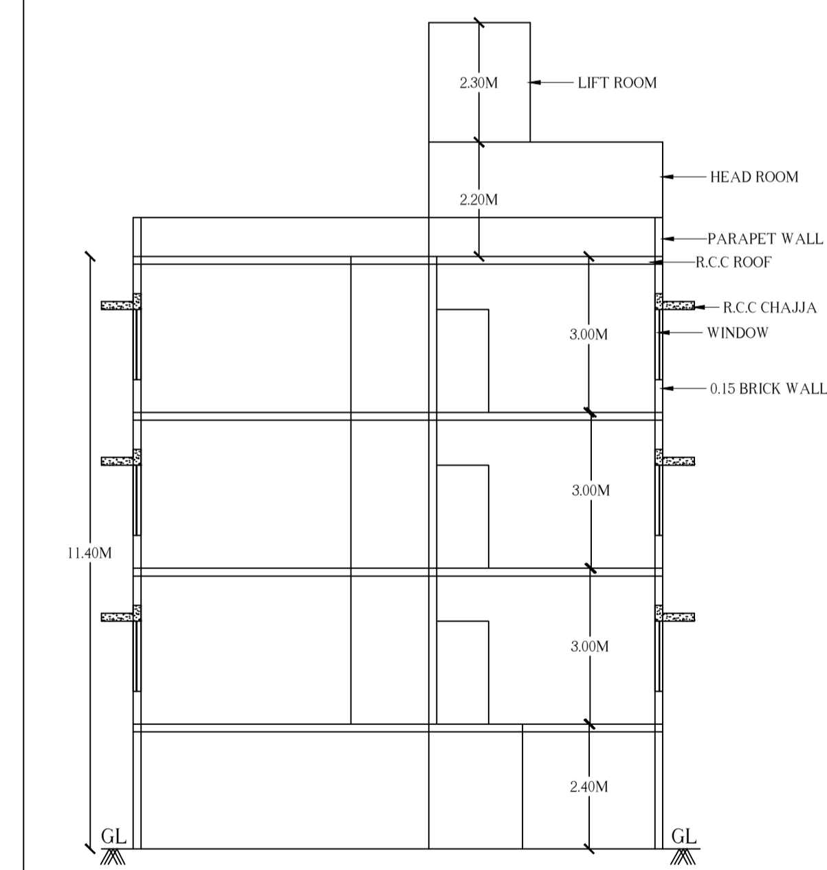
SECTION A-A
